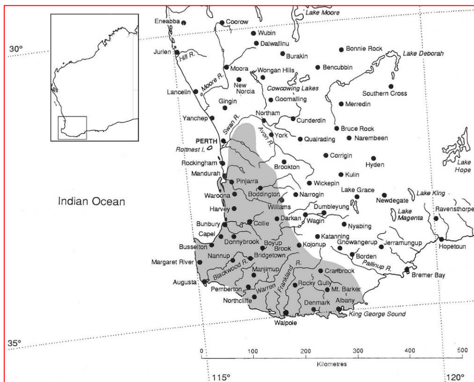
Actual distribución en sur-Oeste del estado Oeste Australiano
